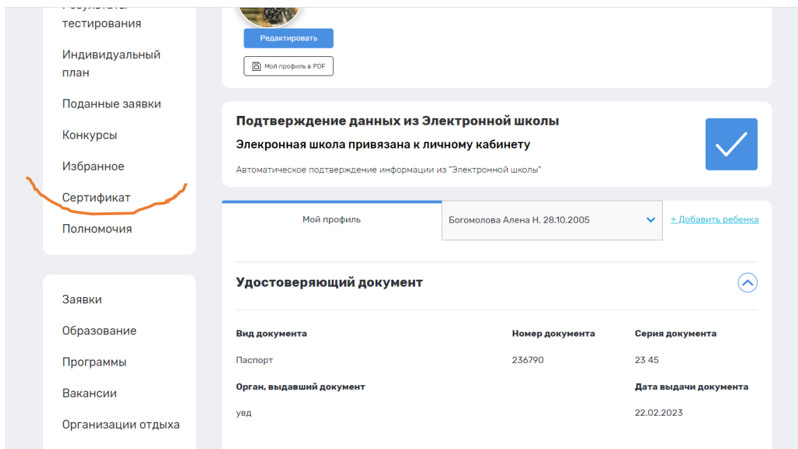
Рис. 7. Кнопка «Сертификат»
